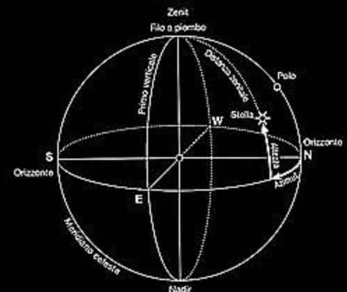
Coordinate Altazimutali
