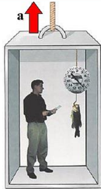
Osservatore 1 in moto acc. = +a
