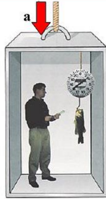
Osservatore 2 in moto acc. = -a
